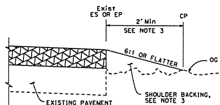
CASE E Vertical Edge
