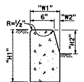
TYPE A1 CURBS See Table A
