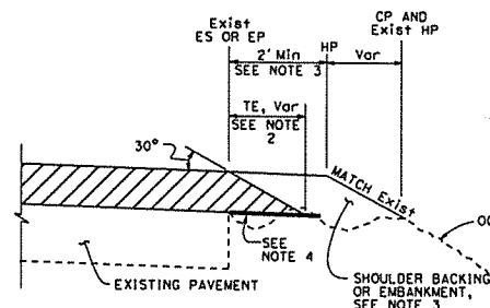
CASE B Tapered Edge
