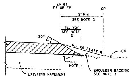
CASE A Tapered Edge
