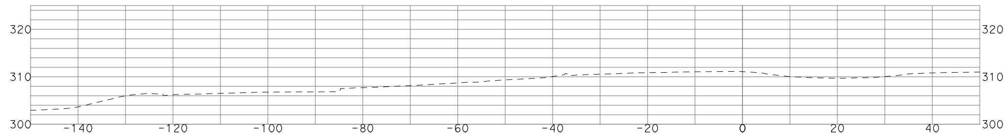
"GSB_R3_SB4" 551+00
